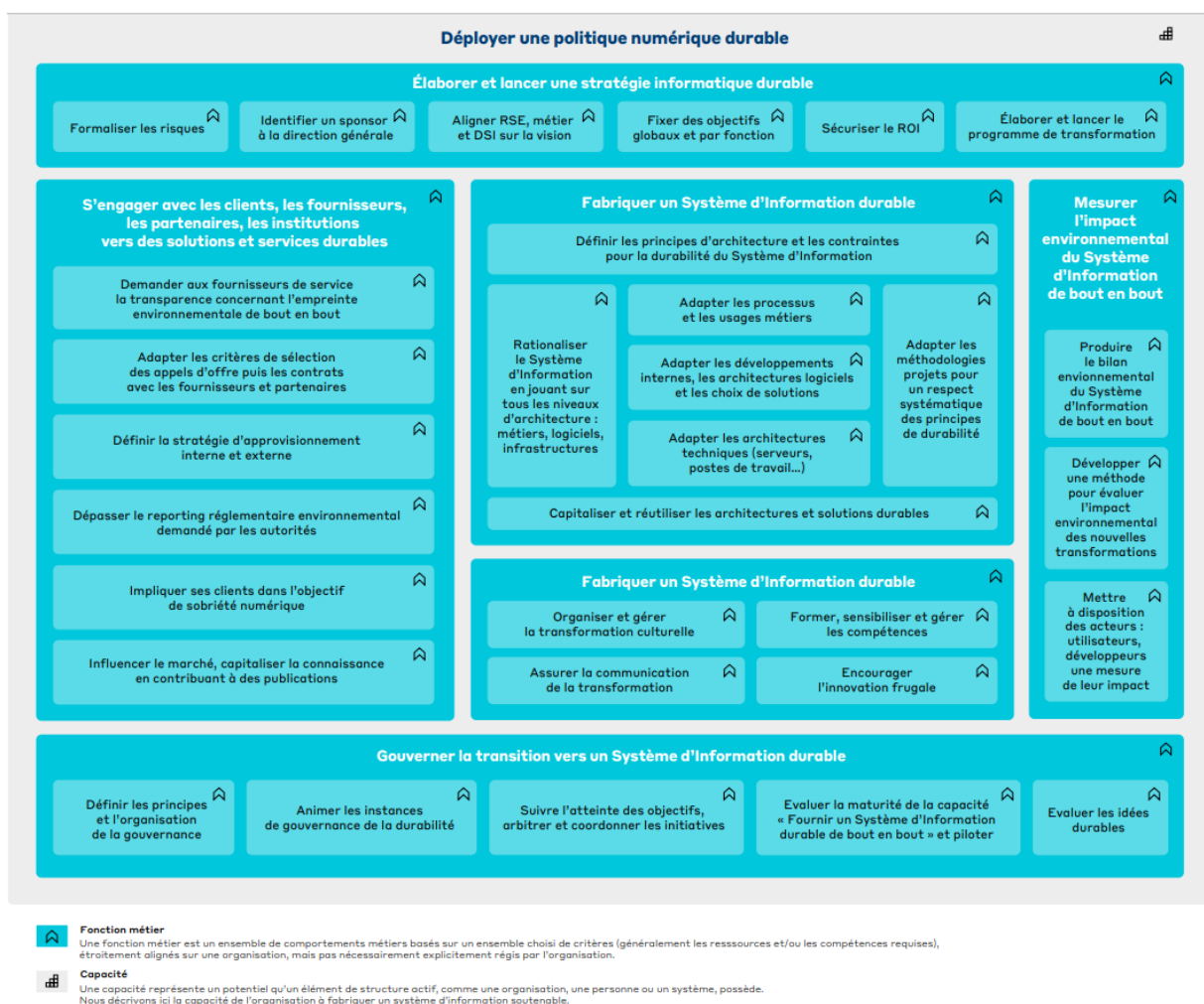
Figure 12 - Modèle de référence – vue détaillée - pour une remise en forme du Système d'Information Source : The Shift Project, production du groupe de travail
