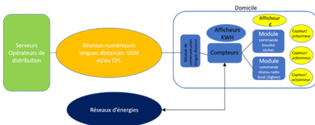
Figure 7 - Architecture du réseau "Compteur communicant". En bleu, modules composant le compteur communicant. Source : The Shift Project, production du groupe de travail
